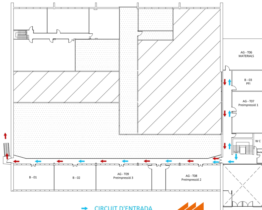
PLANTA PRIMERA
